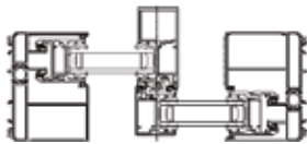
Coupe horizontale du système testé
